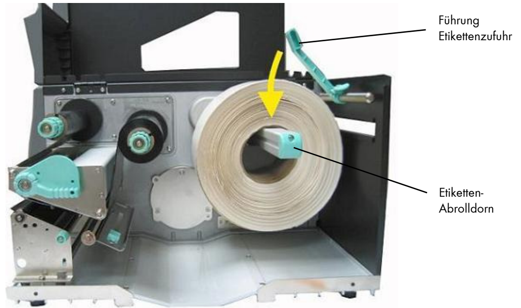
Abb. 5.2.1.e Materialrolle einlegen
