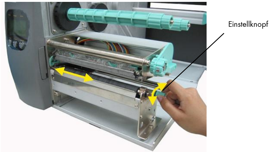
Abb. 5.2.1.k Sensorposition verstellen
