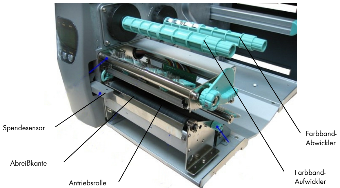
Abb. 2.4.d Detailaufnahme Druckmechanik
