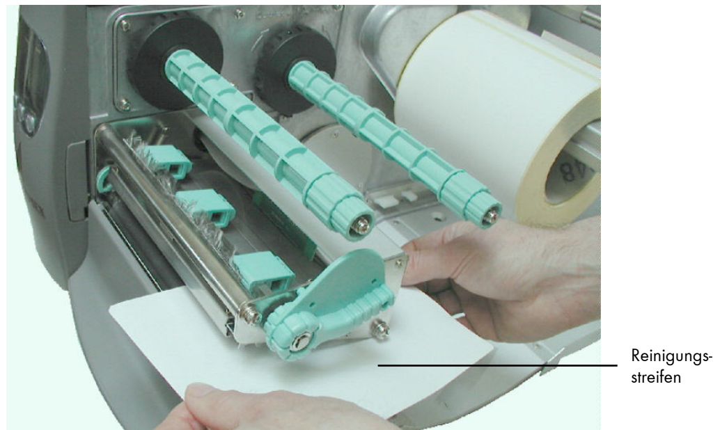
Abb. 9.1.2.b Druckkopf mit Reinigungstreifen reinigen
