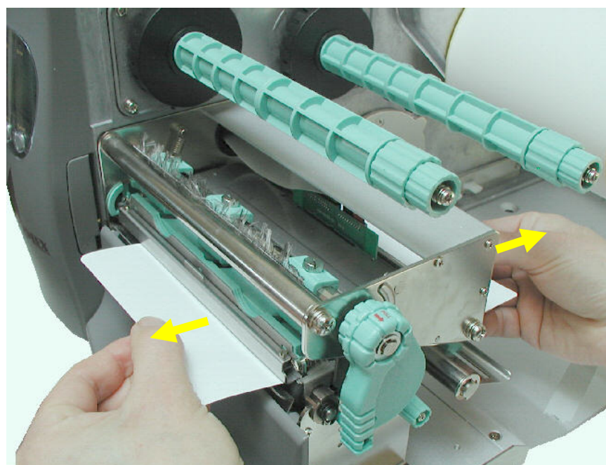
Abb. 9.1.2.c Reinigungstreifen hin- und herbewegen
