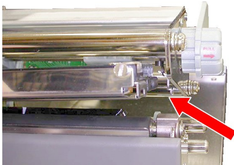
Abb. 9.2.1.d Druckkopf in seitliche Führungen einführen
