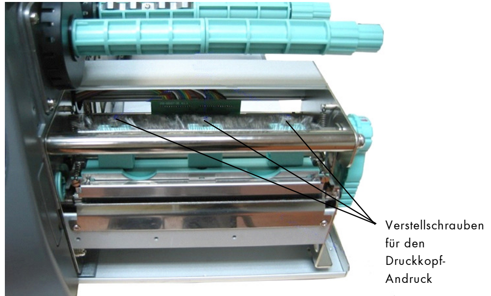
Abb. 5.4.f Druckkopf-Andruckkraft einstellen
