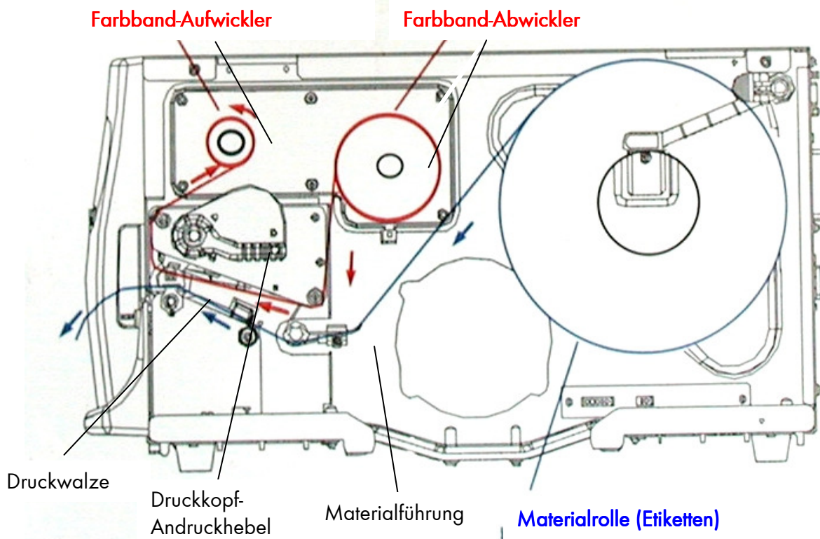
Abb. 5.1.a Material- und Folienverlauf (hier: Tinte auf der Innenseite der Rolle)
