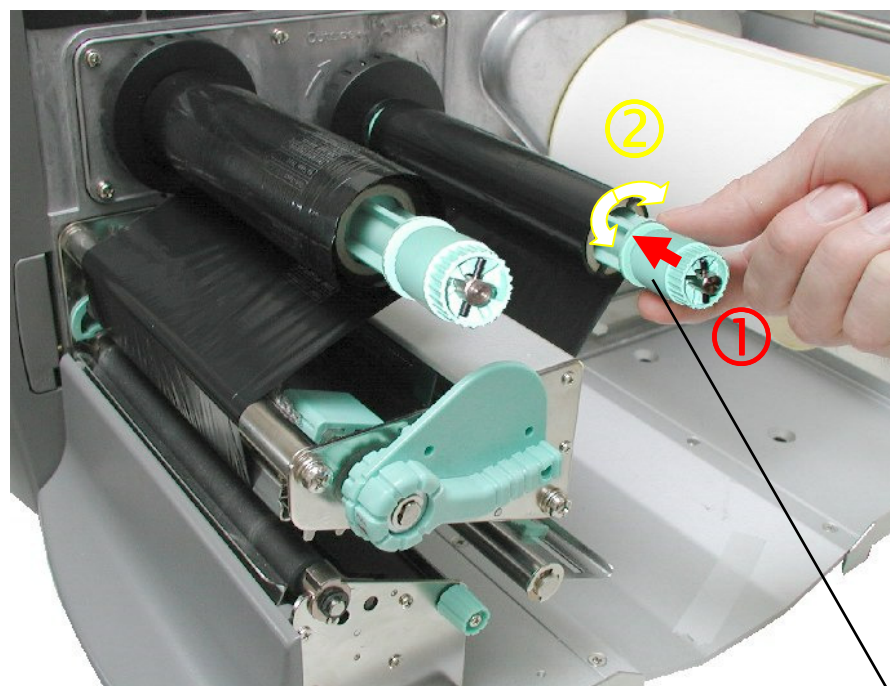
Abb. 5.3.2.a Farbbandspannung justieren
