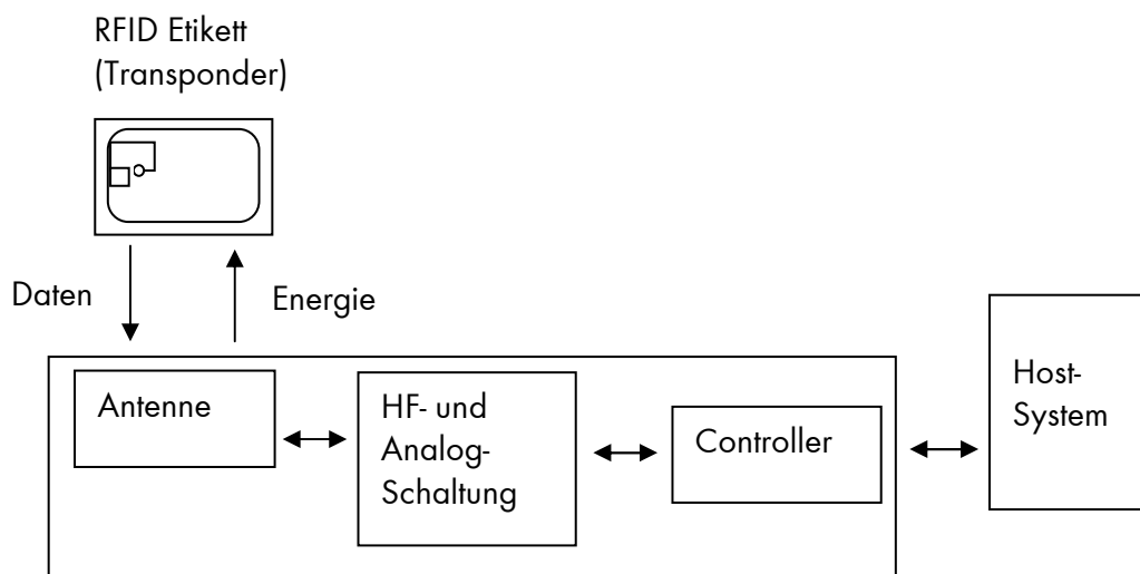
Abb. 1.2.a Blockdiagramm zur Hochfrequenz-Identifikationstechnologie (RFID)
