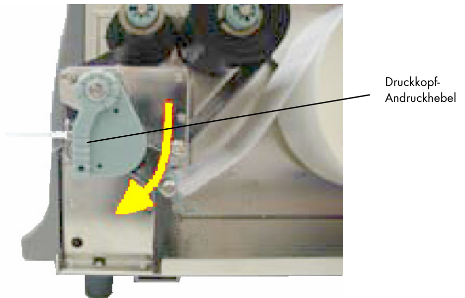
Abb. 5.3.1.f Andruckhebel verriegeln
