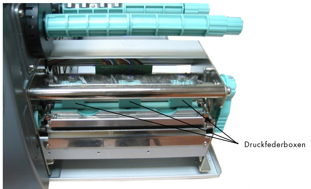
Abb. 5.4.a Druckkopf-Andruck: Position der Druckfederboxen
