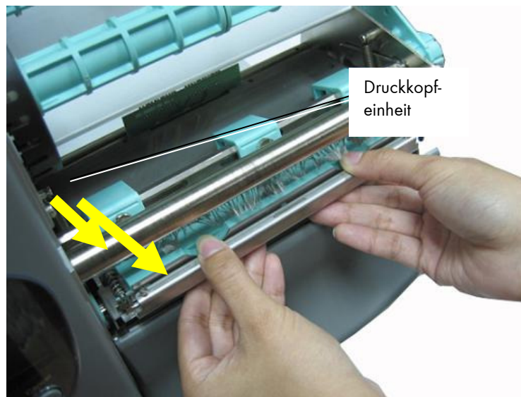
Abb. 9.2.1.b Druckkopf vorsichtig etwas ziehen
