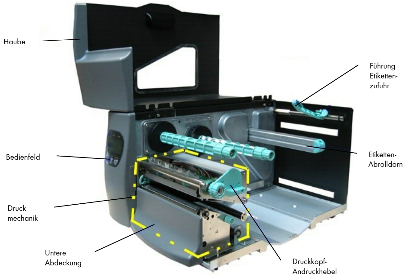
Abb. 2.4.c Drucker geöffnet
